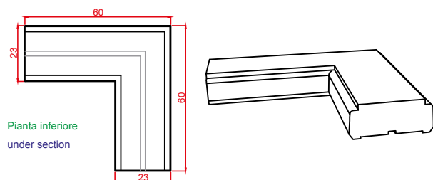
ART. 1255 CORRIMANO GRANDE ANGOLARE h cm 9,5x23 - lunghezza cm 60+60 - peso kg 33 3.74' 'x9.05' ' tall - 23.62' ' +23.62' ' lenght - 72.75 lbs
