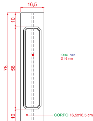
ART. 1273 PIANTINO INTEGRATO GRANDE h cm 78 - peso kg 38 30.70' ' tall - 83.77 lbs
