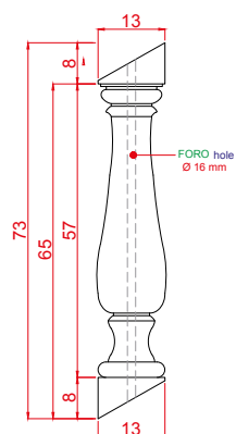
ART. 1231 COLONNETTA SIRMIONE II PER SCALA h cm 73 - peso kg 15 28.74' ' tall - 33.06 lbs
