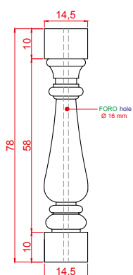
ART. 1236 COLONNETTA BONIFACIO h cm 78 - peso kg 22 30.70' ' tall - 48.50 lbs
