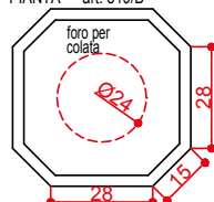
PIANTA art. 819/B
