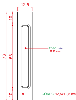
ART. 1272 PIANTINO INTEGRATO PICCOLO h cm 73 - peso kg 24 28.74' ' tall - 52.91 lbs
