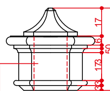
PROSPETTO art. 819/E
