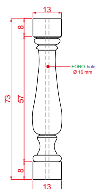
ART. 1230 COLONNETTA SIRMIONE II h cm 73 - peso kg 16 28.74' ' tall - 35.27 lbs
