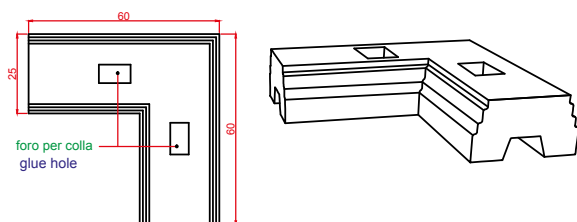
ART. 1215 BASE GRANDE ANGOLARE h cm 14x25 - lunghezza cm 60+60 peso kg 49 5.51' 'x9.84' ' tall - 23.62' ' +23.62' ' lenght - 108 lbs
