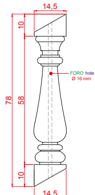
ART. 1237 COLONNETTA BONIFACIO PER SCALA h cm 78 - peso kg 20 30.70' ' tall - 44.09 lbs
