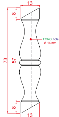
ART. 1233 COLONNETTA BORBONE PER SCALA h cm 73 - peso kg 16 28.74" tall - 35.27 lbs
