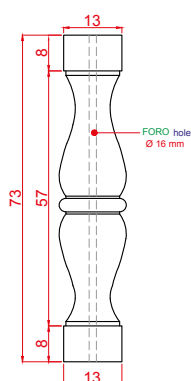
ART. 1232 COLONNETTA BORBONE h cm 73 - peso kg 17 28.74" tall - 37.47 lbs
