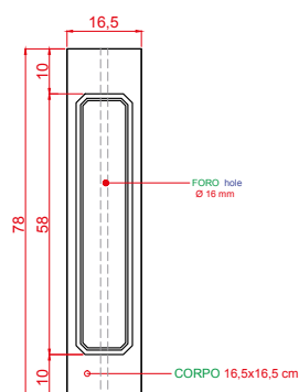
ART. 1273 PIANTINO INTEGRATO GRANDE h cm 78 - corpo cm 16,5x16,5 peso kg 38 30.70" tall - 6.49" L - 6.49" W - 83.77 lbs
