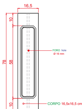
ART. 1273 PIANTINO INTEGRATO GRANDE h cm 78 - corpo cm 16,5x16,5 peso kg 38 30.70" tall - 6.49" L - 6.49" W - 83.77 lbs
