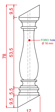
ART. 1239 COLONNETTA SAVOIA PER SCALA h cm 78 - peso kg 27 30.70" tall - 59.52 lbs
