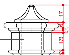
PROSPETTO art. 819/E
